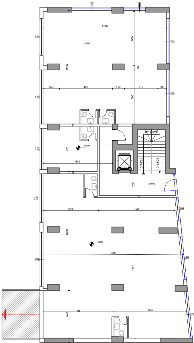
PLANIMETRIA SH 1: 200
